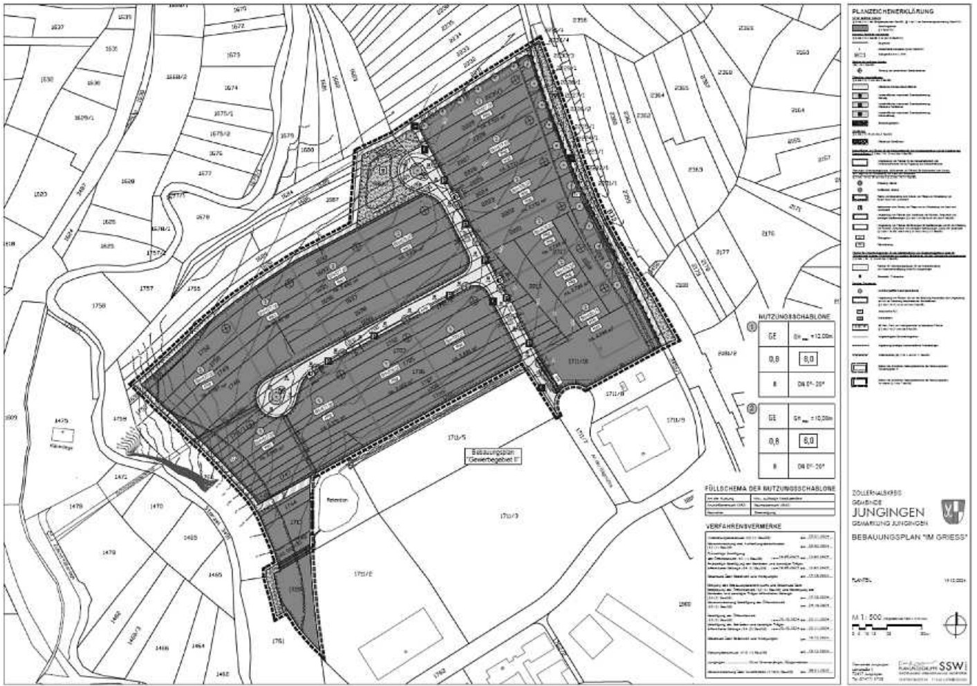
Lageplan des Bebauungsplans „Im Griess“, Planungsgruppe SSW GmbH, Ludwigsburg, vom 19.12.2024
